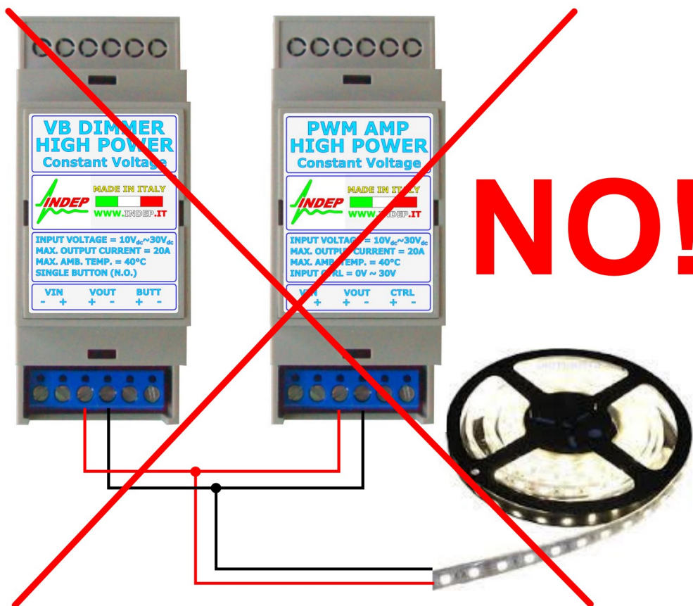
Figura4. Le uscite dei dispositivi non vanno poste in parallelo.
