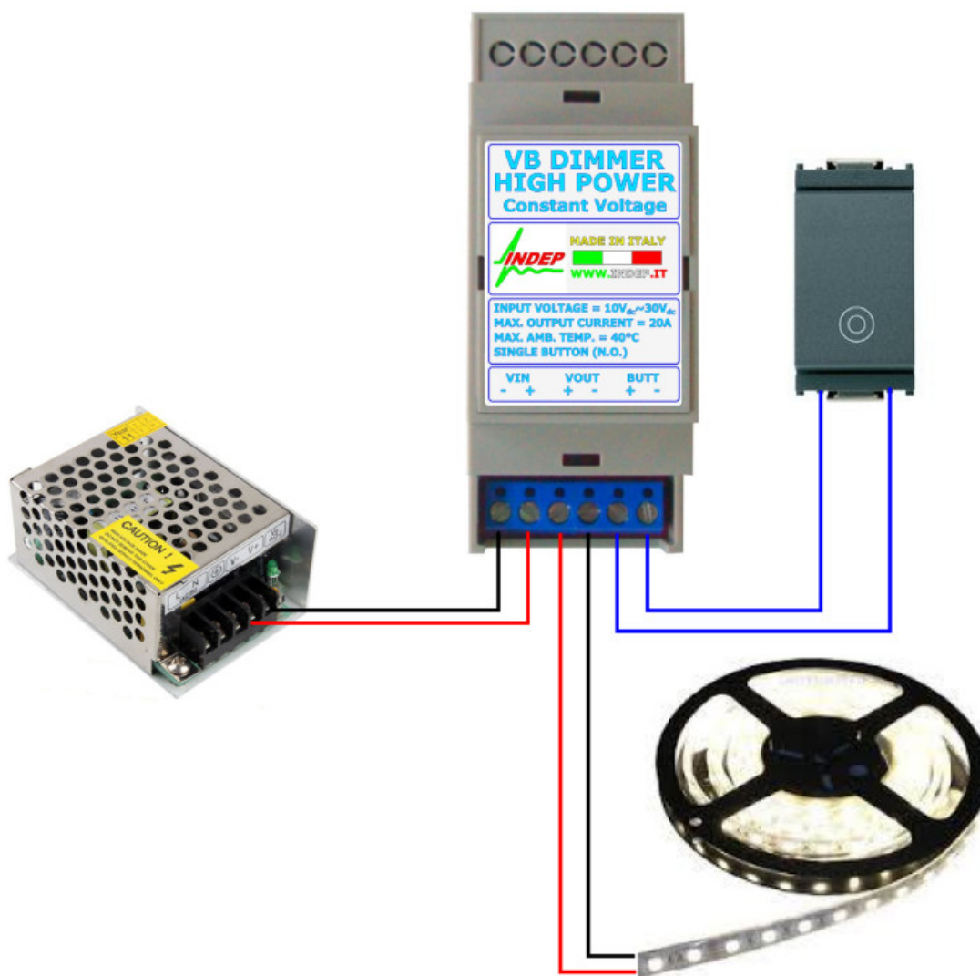
Figura2. Schema dei collegamenti.
