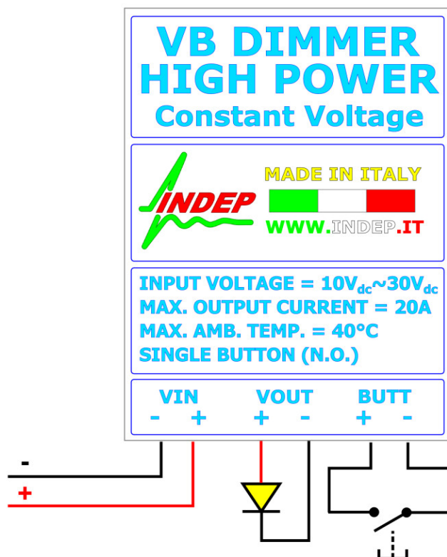
Figura1. Schema elettrico: linea di alimentazione, carico, pulsante.
