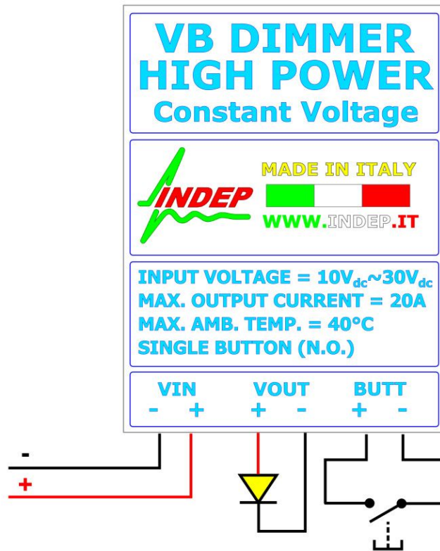
Figura1. Schema elettrico: linea di alimentazione, carico, pulsante.
