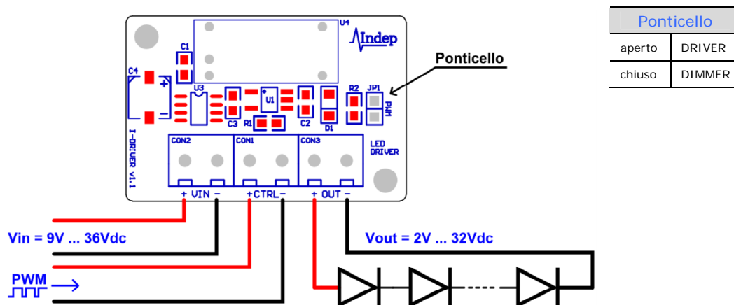
Fig.2: Configurazione Dimmer a modulazione di corrente: 0%...100%. Controllo PWM in tensione, ponticello inserito.
