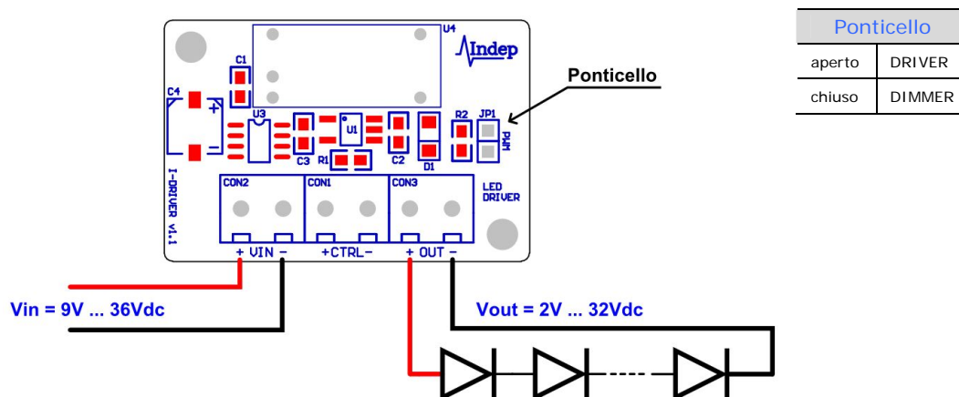
Fig.1: Configurazione Driver a corrente costante. Ponticello tolto (aperto). Solo su richiesta.
